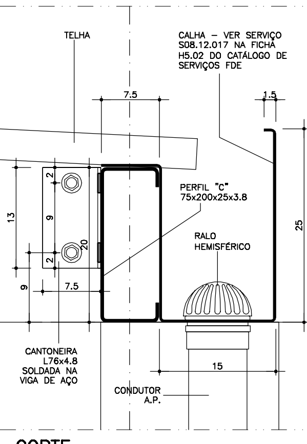
CORTE TRANSVERSAL A TERÇA
