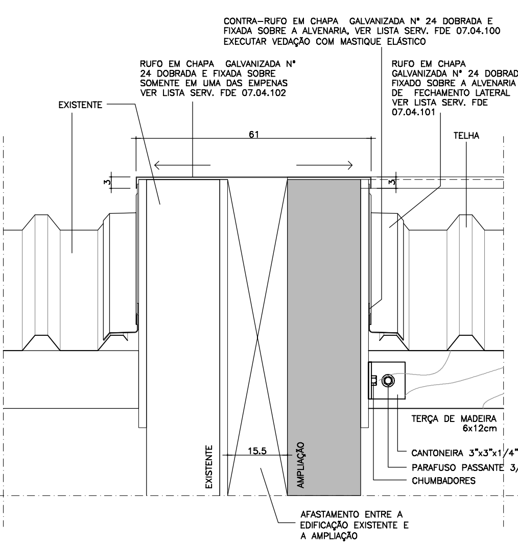
CORTE LONGITUDINAL A TERÇA
