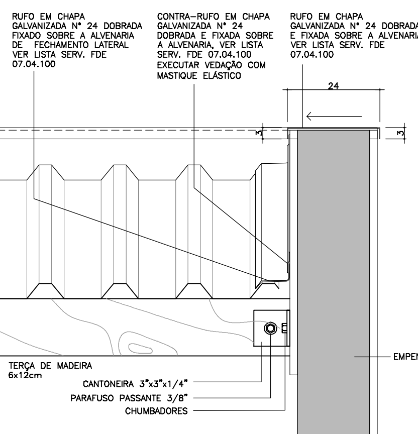
CORTE LONGITUDINAL A TERÇA
