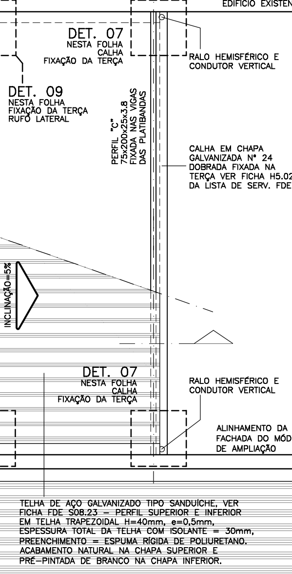
CORTE TRANSVERSAL A TERÇA
