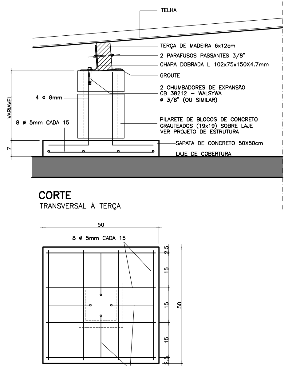
PLANTA SAPATA ARMAÇÃO
