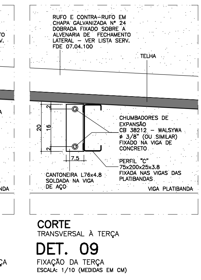
CORTE TRANSVERSAL A TERÇA
