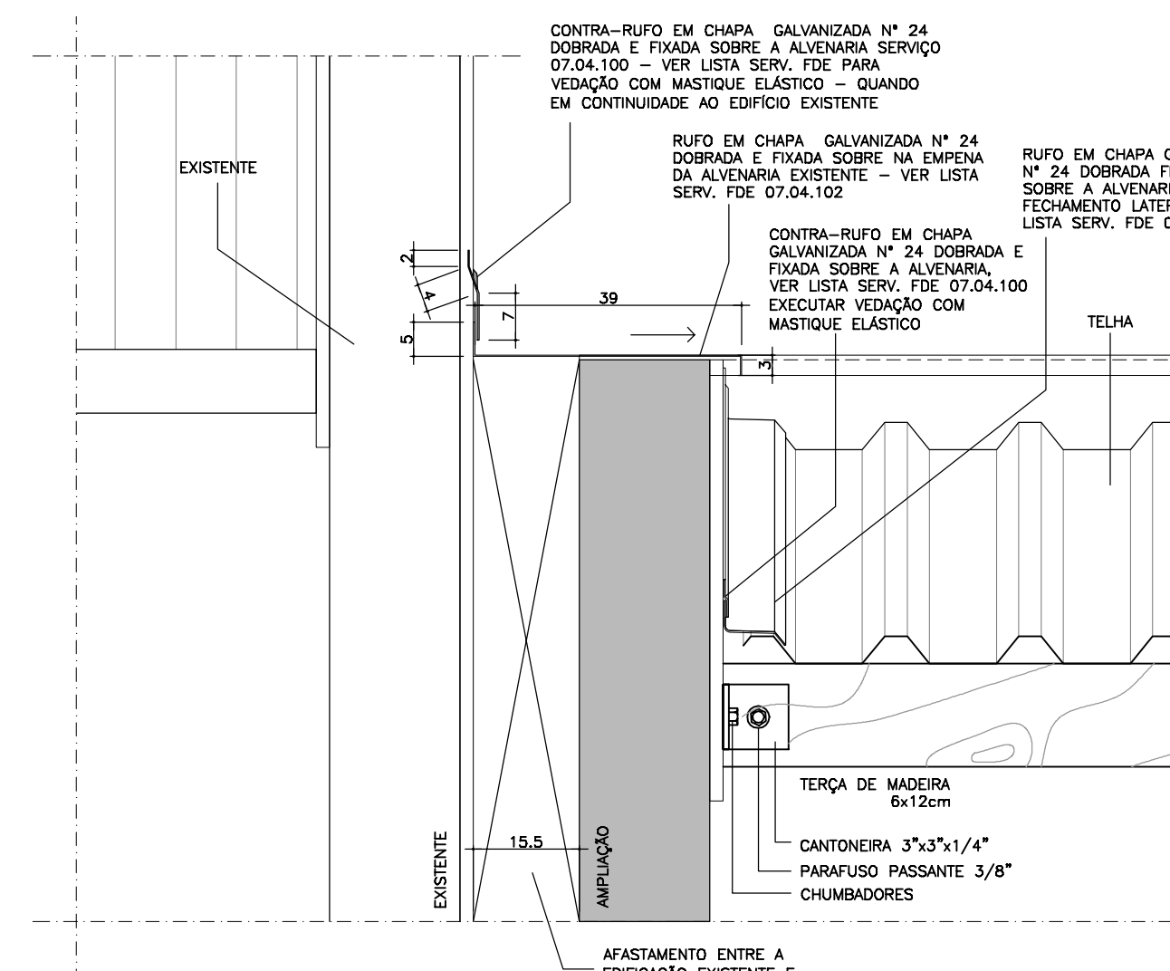
CORTE LONGITUDINAL A TERÇA
