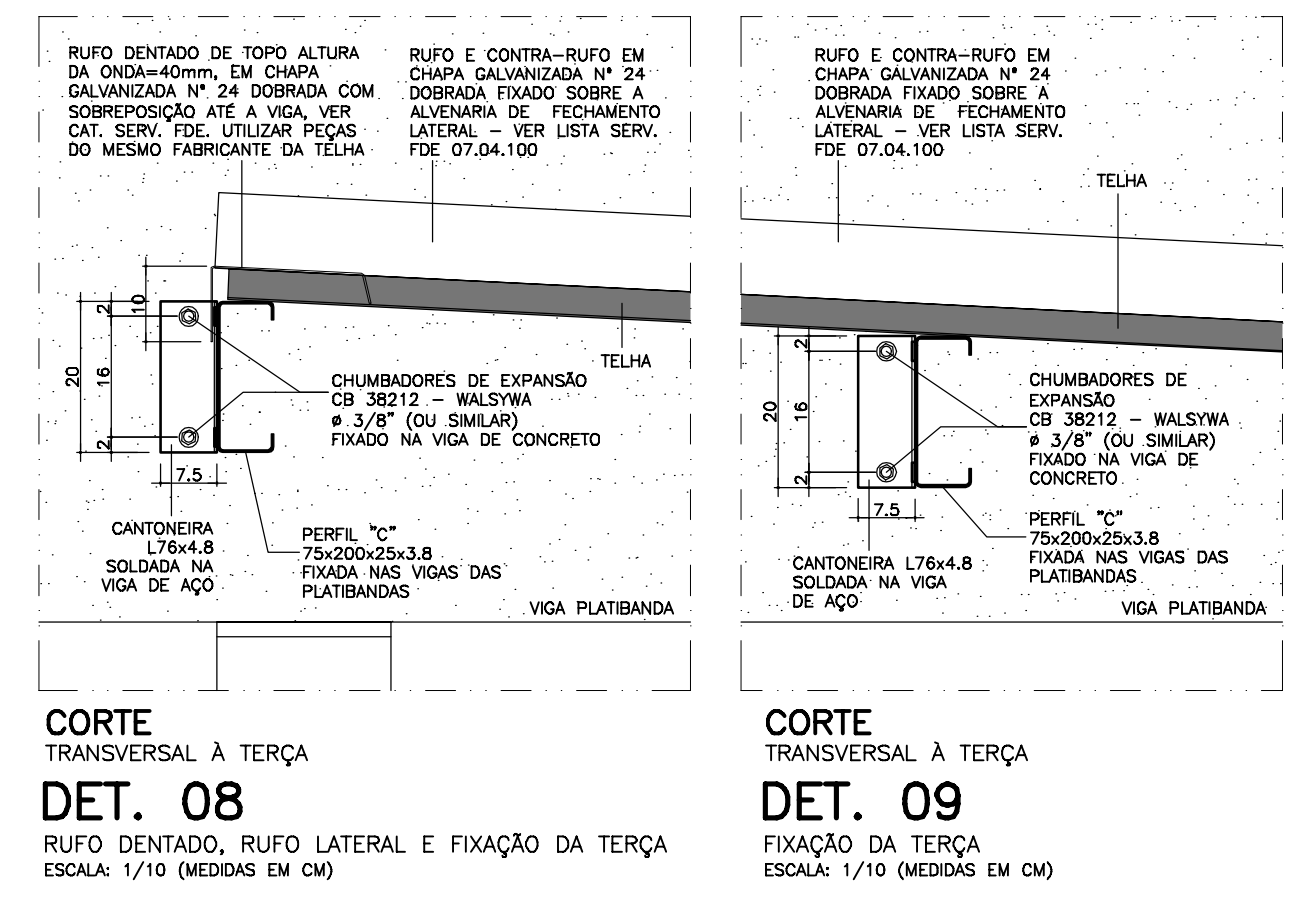
CORTE TRANSVERSAL A TERÇA
