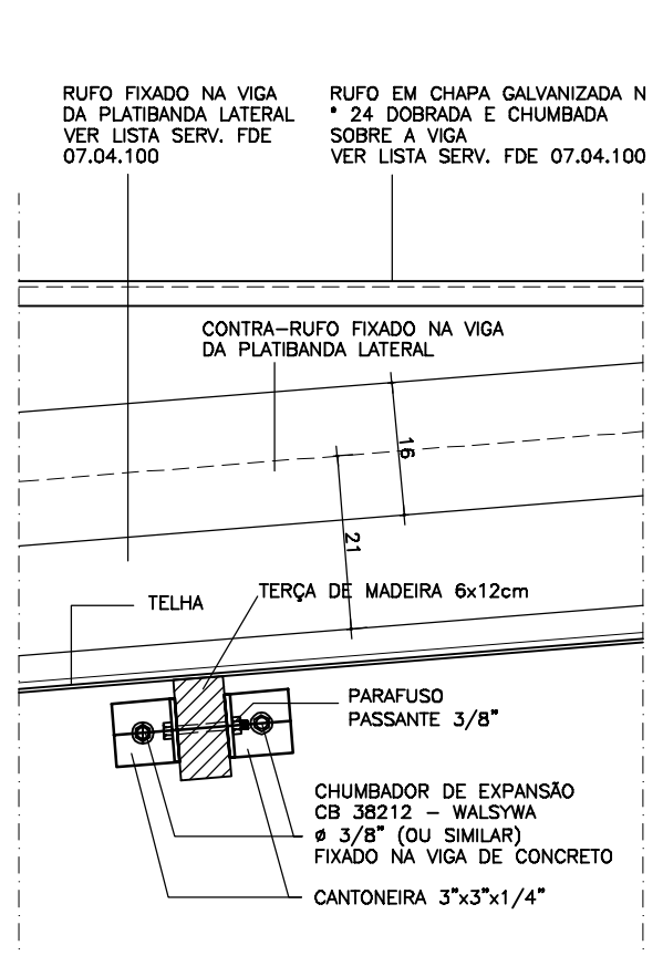
CORTE LONGITUDINAL A TERÇA
