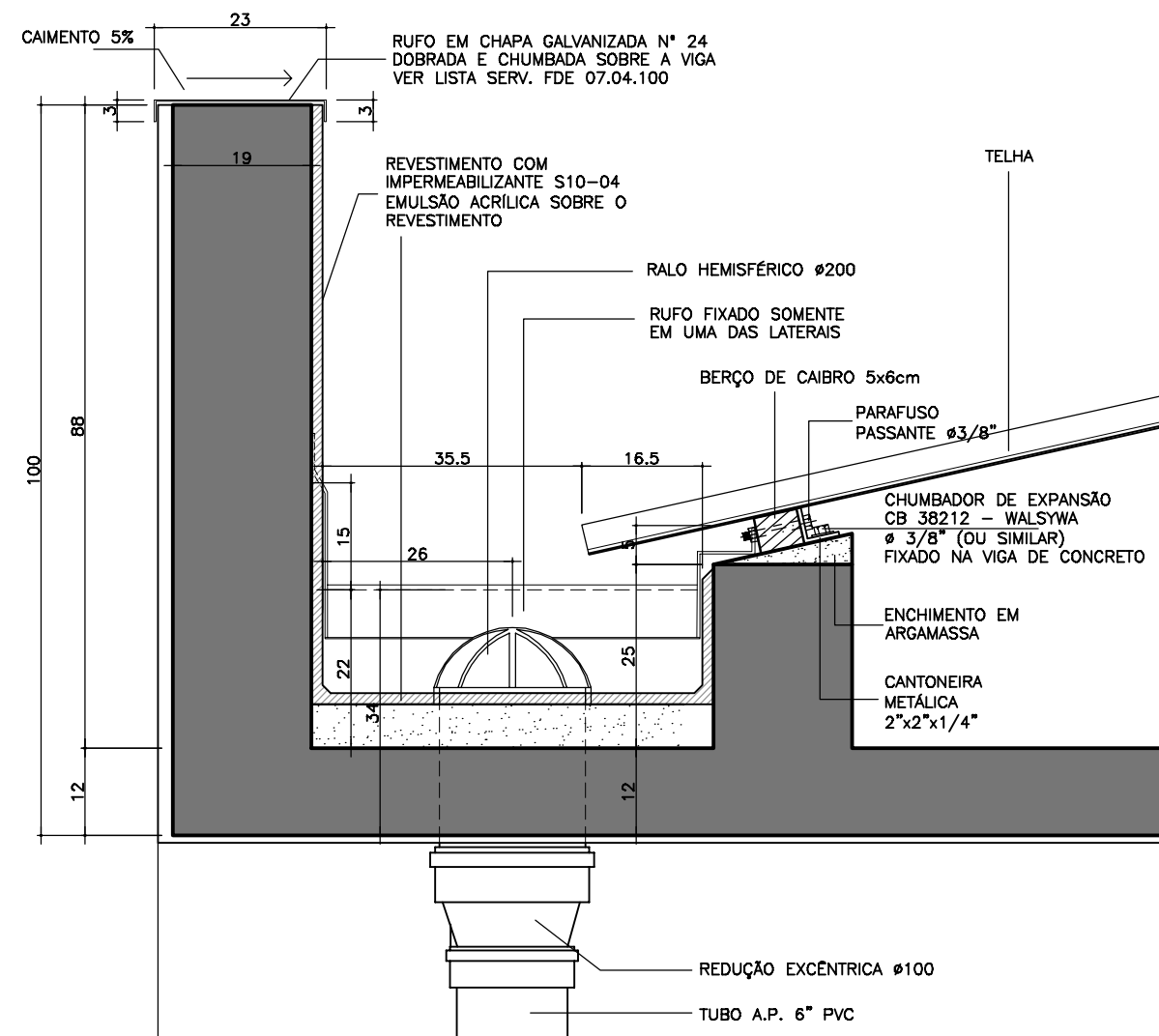
CORTE LONGITUDINAL A TERÇA
